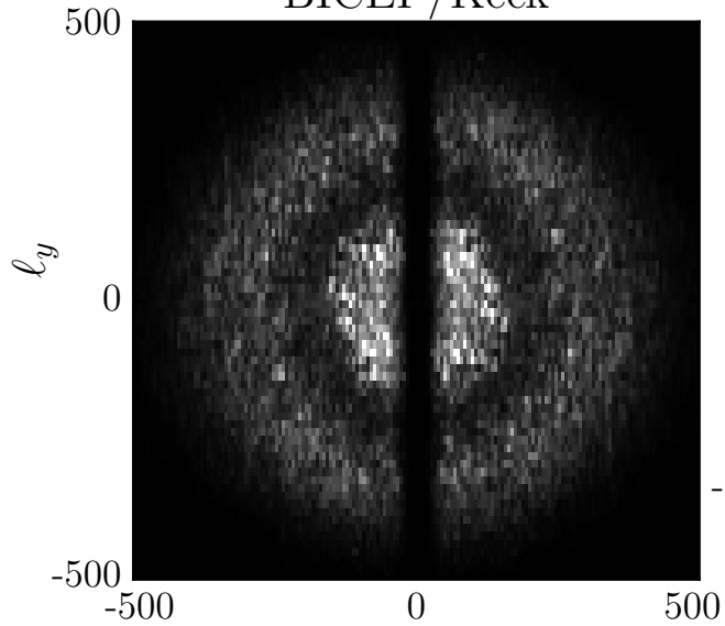
BICEP/Keck
