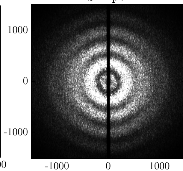
SPTpol
